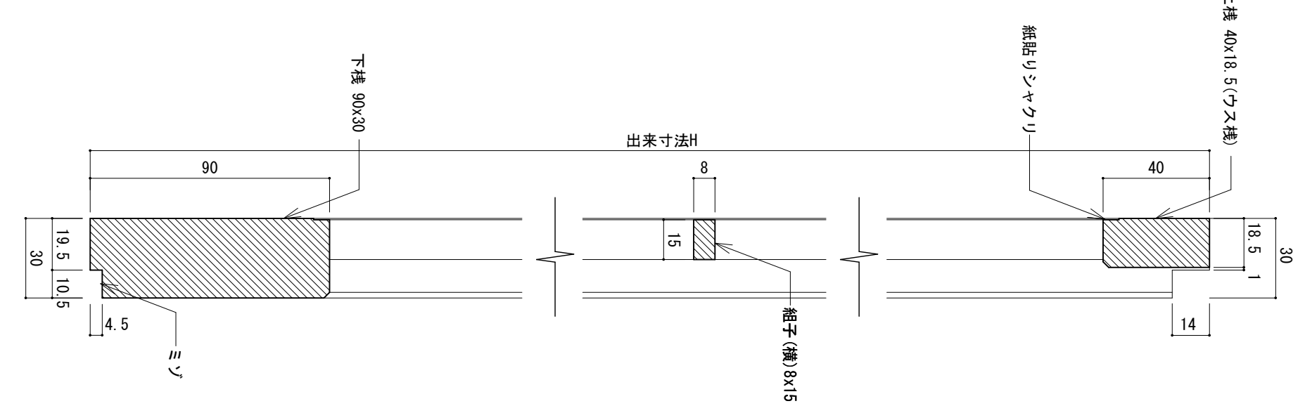
縦断面詳細図 S:1/2
