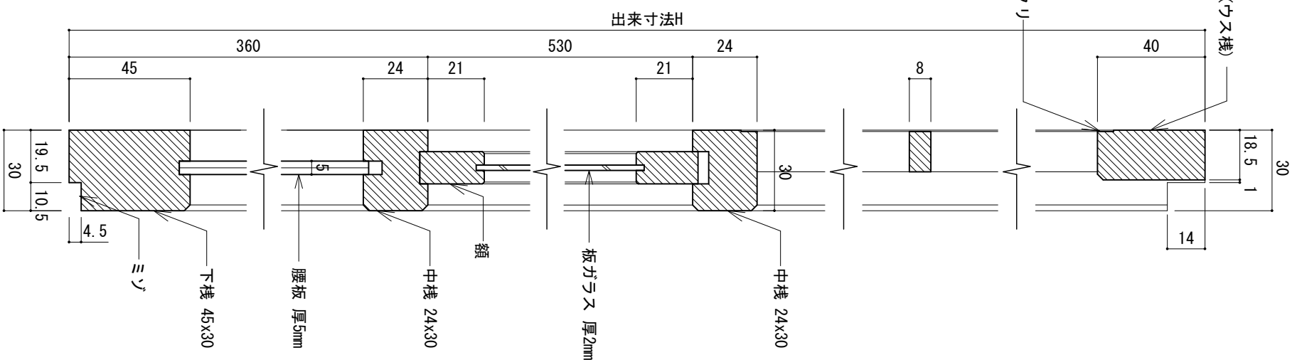
縦断面詳細図 S:1/2
