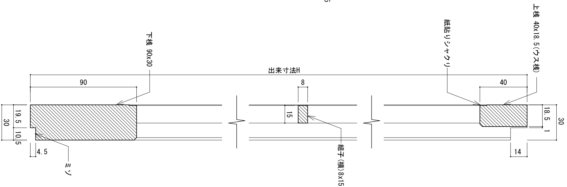
縦断面詳細図 S:1/2
