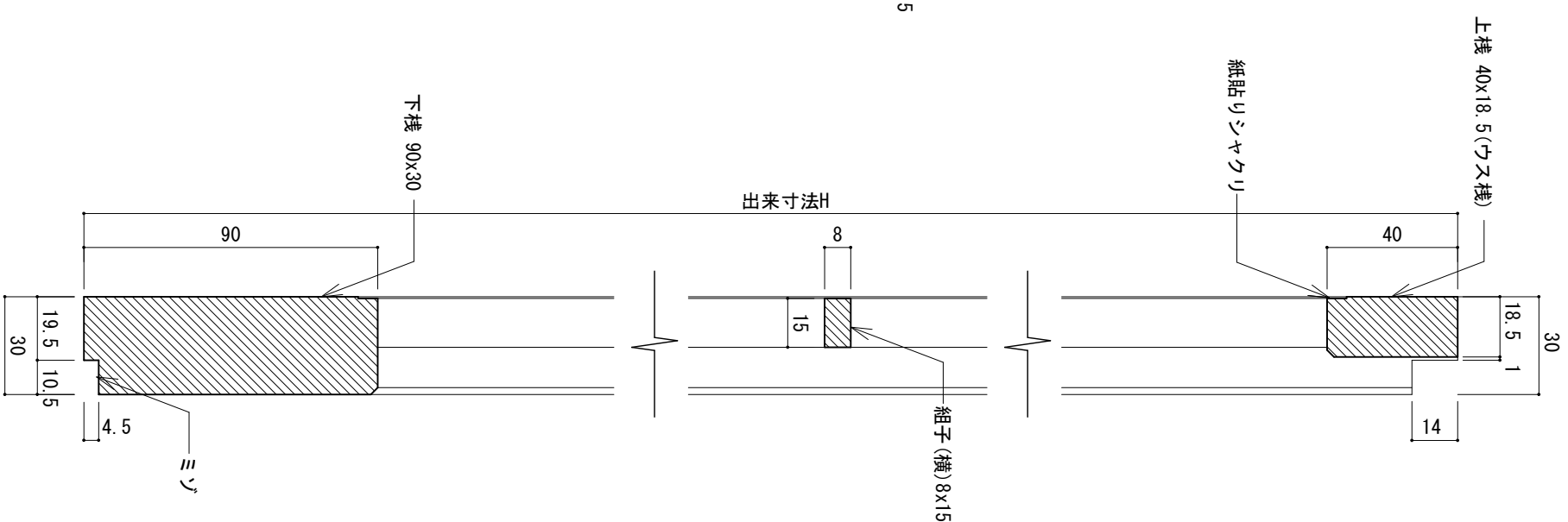
縦断面詳細図 S:1/2
